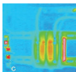
設備温度計測
