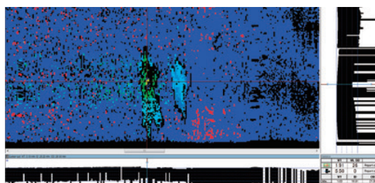
水浸法超音波探傷試験チューブ探傷画面
