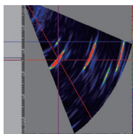
フェーズドアレイ法超音波探傷試験
