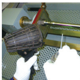
軸通電法による磁気探傷試験
