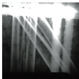
コンクリート内部の鉄筋配管位置
